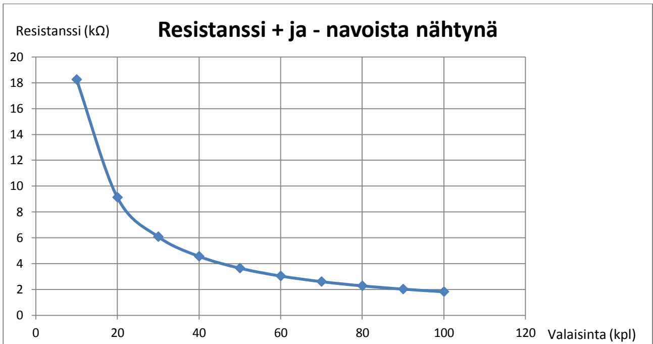
Kuvaaja 1.1 ESC-200 –keskus, yhden väylän resistanssi valaisinten kappalemäärän mukaan
